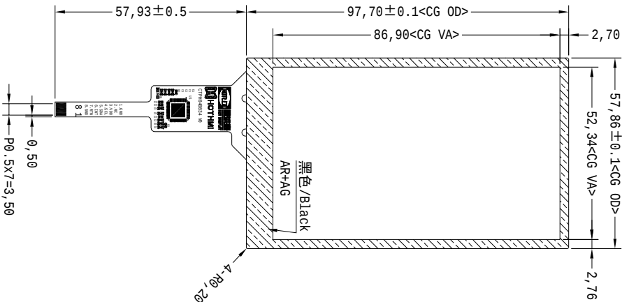
正视图 Front view
